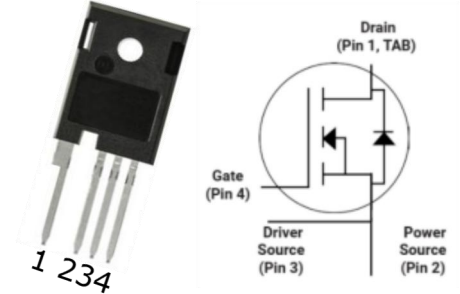
TO-247-4L
